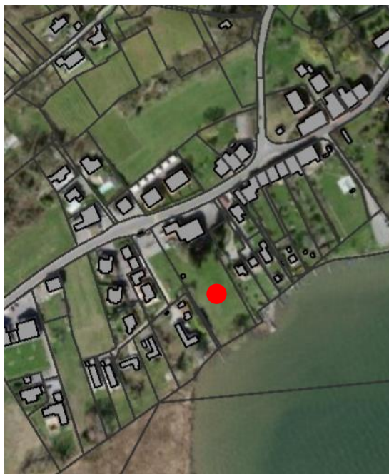
Plan de situation, échelle 1:5'000
