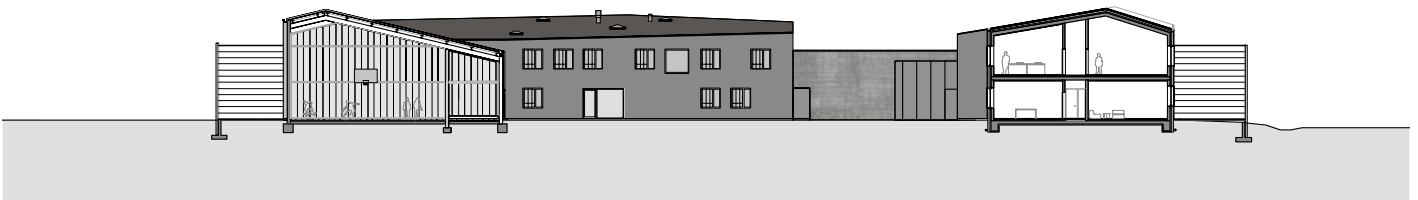
coupe B-B
