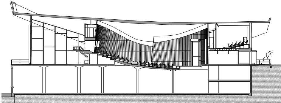
Coupe longitudinale Auditorium
