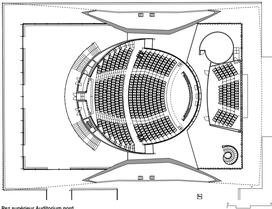
Rez supérieur Auditorium nord
